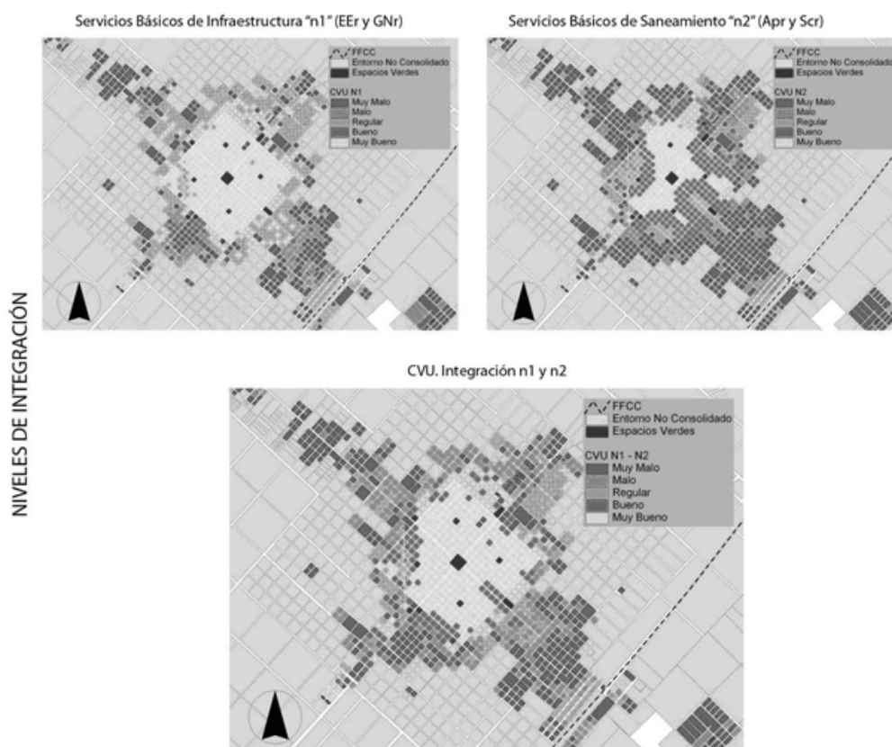
Figura 84. Índices de CVU. Diferentes niveles de integración.
