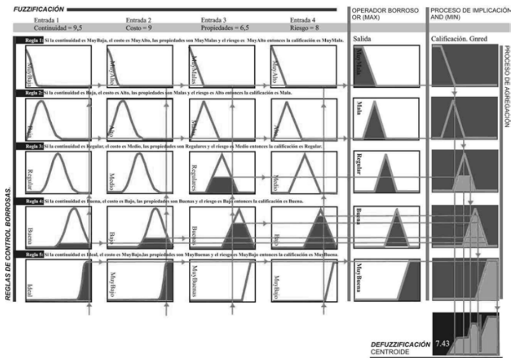
Figura 13. Diagrama de inferencia borroso.
