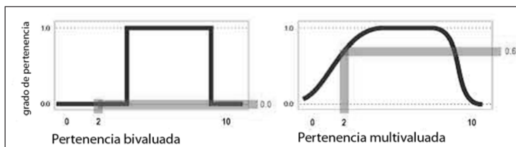
Figura 8. Conjunto NO Borroso – Conjunto Borroso.
