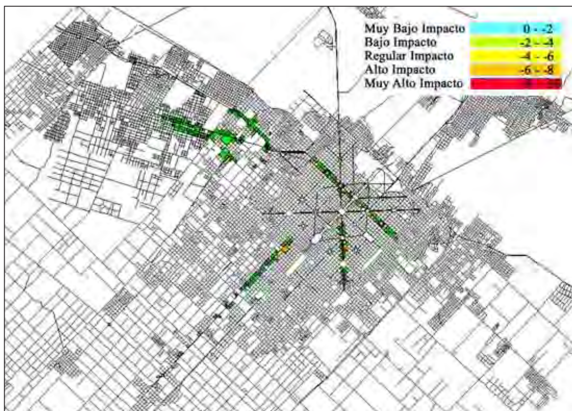
Perfil de CVU de Contaminación de Aire.
